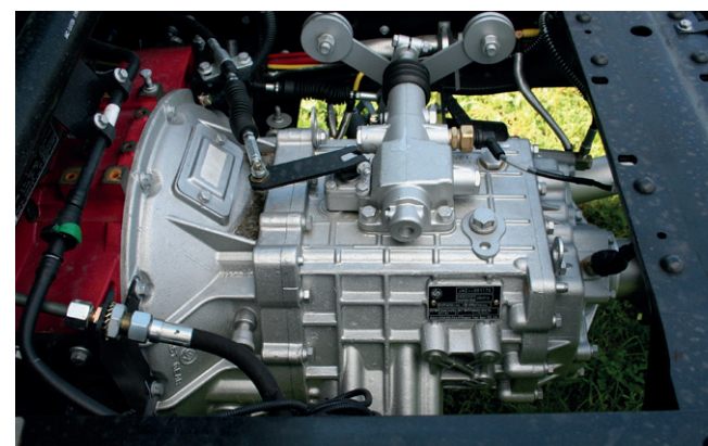
Шестиступенчатая механическая коробка передач 6DS60T-D – китайского производства
